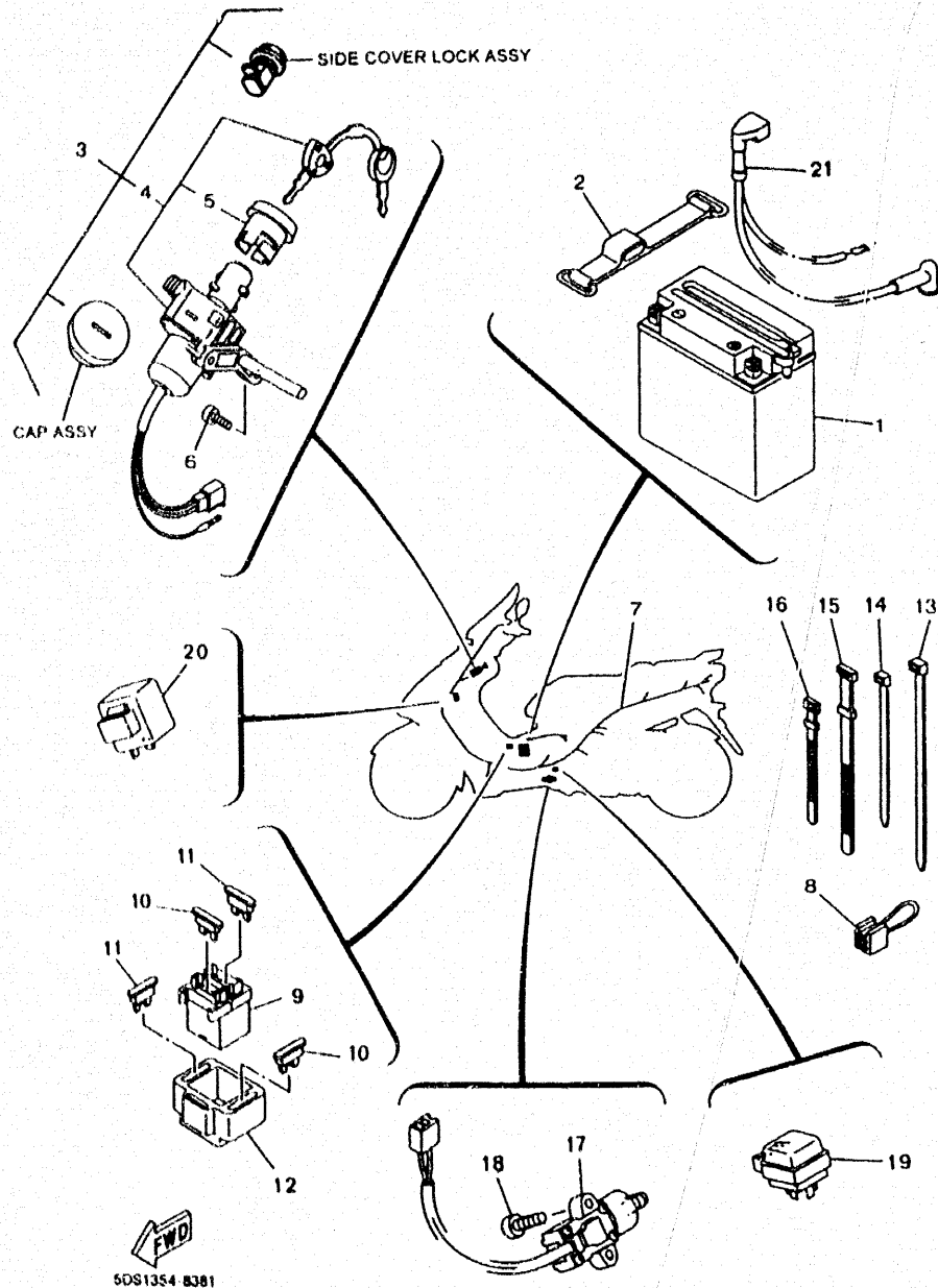
FIG. 38 - GRUPO ELECTRICO 2
