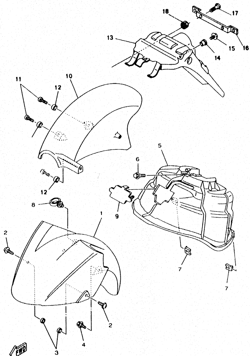
FIG. 17 - FRONTAL DELANTERO
